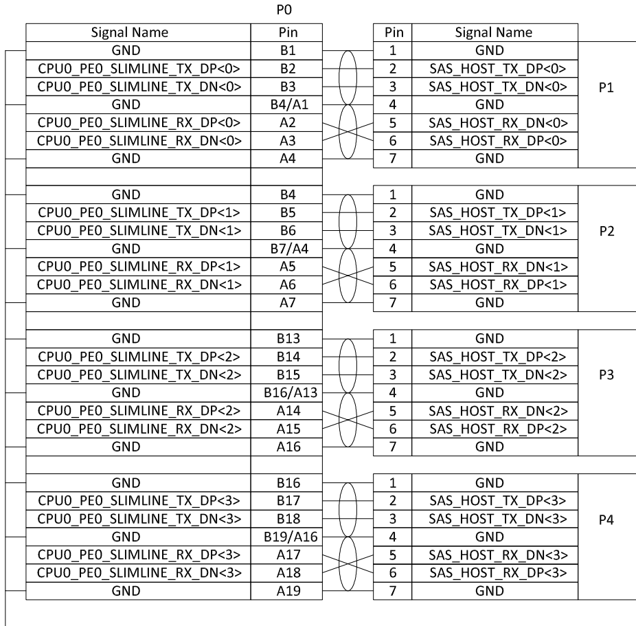
WIRING TABLE
